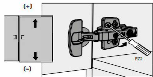
Эксцентриковая регулировка по высоте
