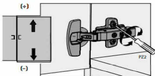
Регулировка по высоте за счет шлицевых отверстий
